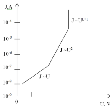
Şəkil 2. İtterbium (Yb) ilə aşqarlanmış \text{Ga}_2\text{Te}_3\langle\text{Yb}\rangle kristalının otaq temperaturunda Volt-ampere xarakteristikası
