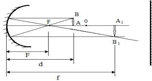
Şəkil 2. Çökük güzgüdə xəyalın qurulması. F – güzgünün fokus məsafəsi; d-cisimdən güzgüyə qədər məsafə, f- güzgüdə xəyala qədər məsafə
